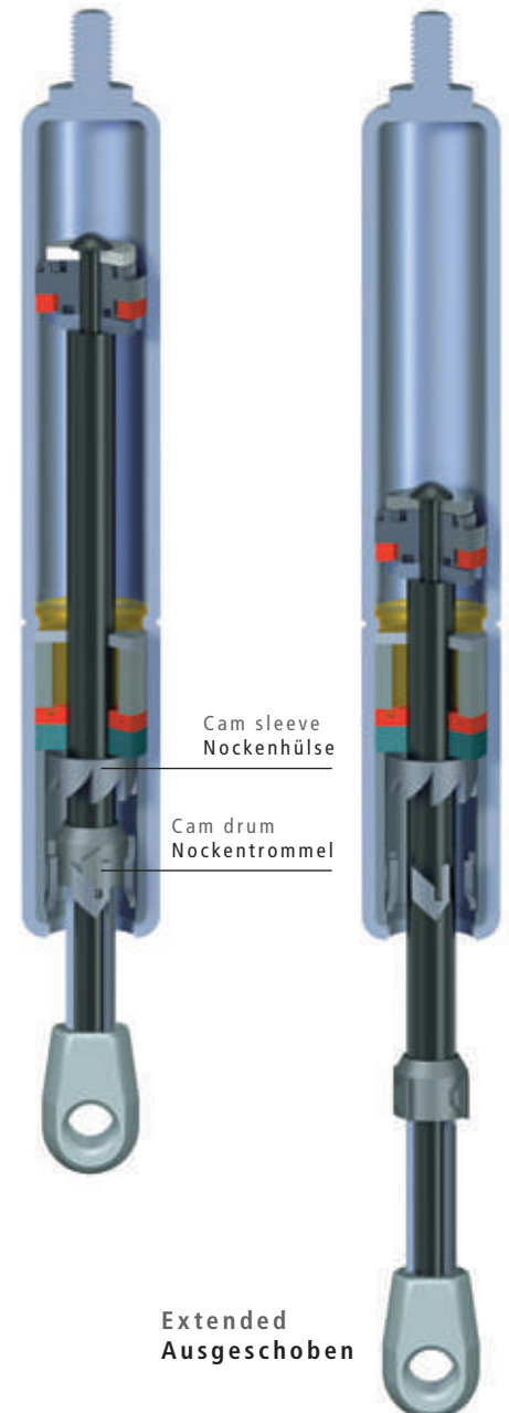
Locked in compressed position Eingeschoben arretiert
